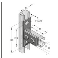
Wspornik z płytką zaciskową poprzeczny
