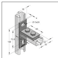
Wspornik z płytką zaciskową wzdłużny
